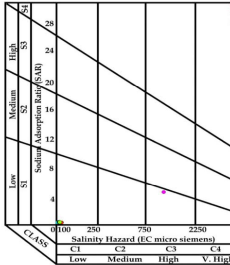
Fig. 3 USSSL diagram – POM
